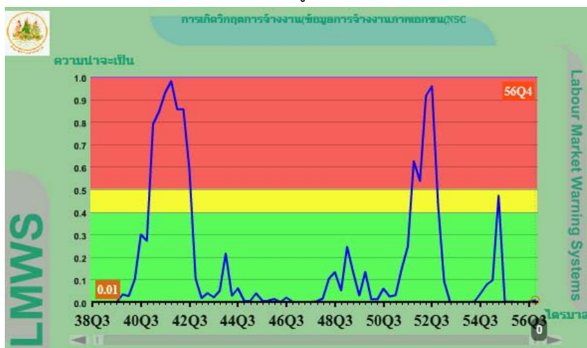
กราฟแสดง ProbitModel ของการจ้างงานNSO
