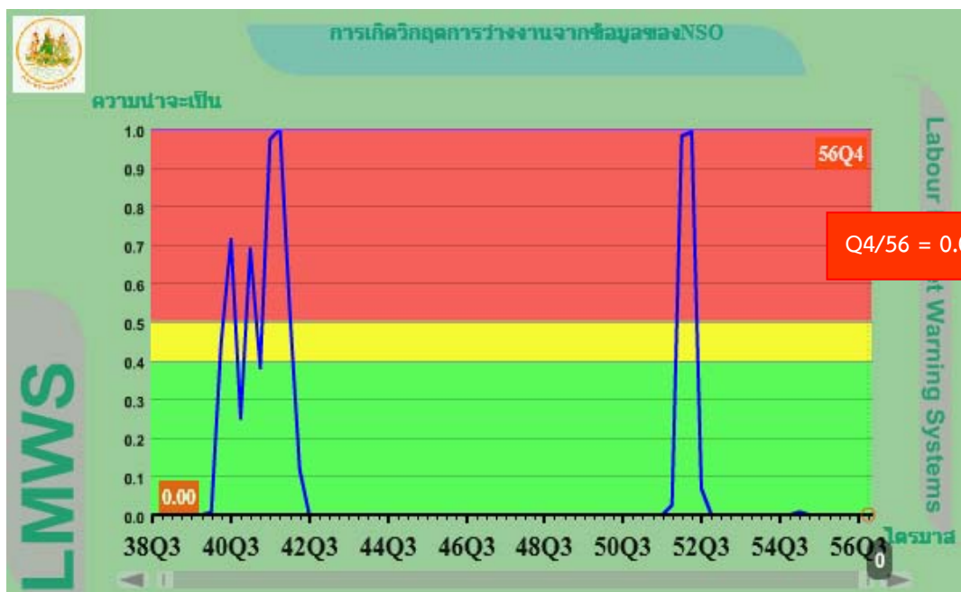
กราฟแสดง ProbitModel ของการว่างงาน
